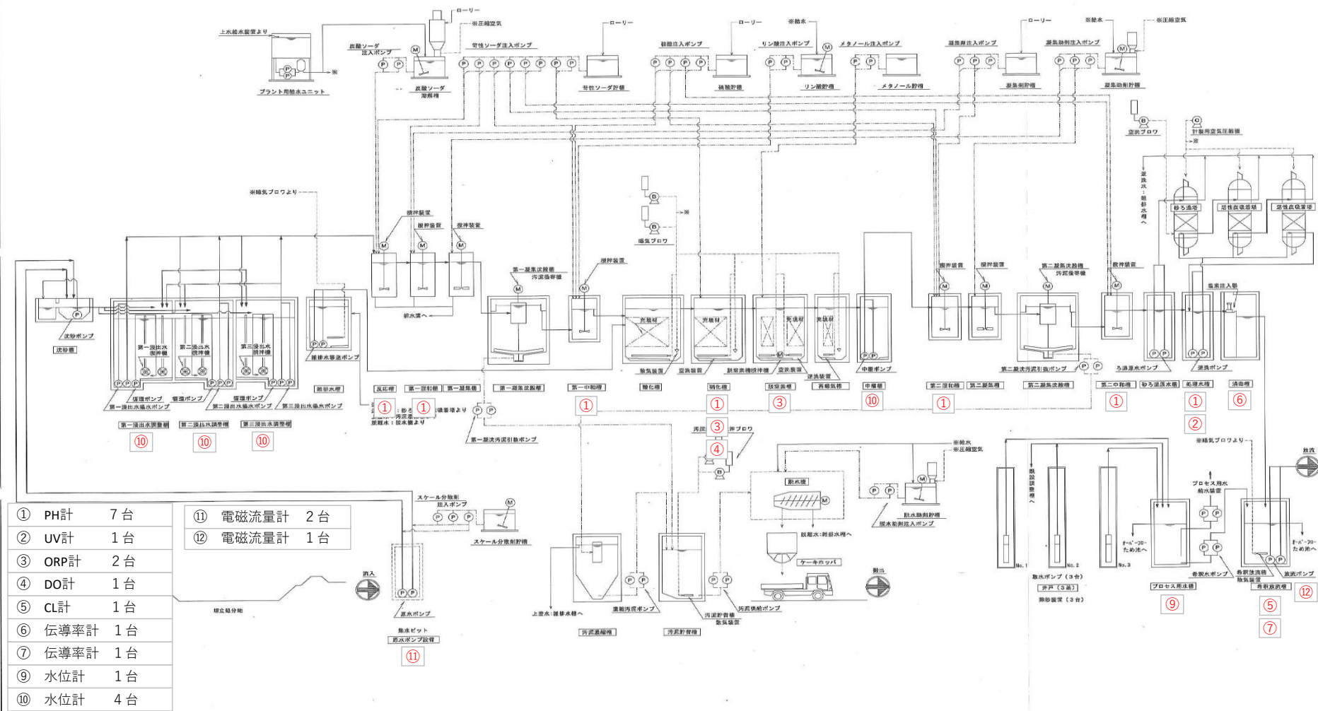
大日向クリーンパーク 水処理フローシート
